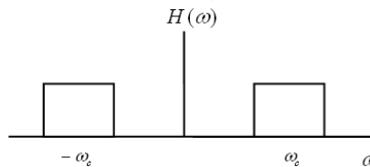
شکل (۲۶-۳): طیف کانال میان گذر (محدوده باند عبور مجاز)
