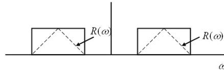
شکل (۲۸-۳): طیف سیگنال پس از انتقال
